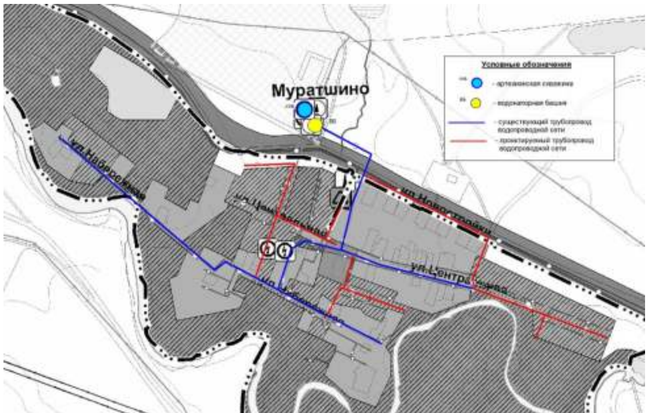
Рисунок 2.4.9.2 – Расположение существующих и перспективных объектов системы водоснабжения с. Муратшино
