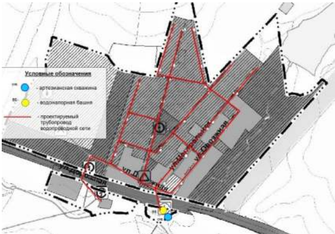
Рисунок 2.4.9.7 – Расположение существующих и перспективных объектов системы водоснабжения п. Бугринка
