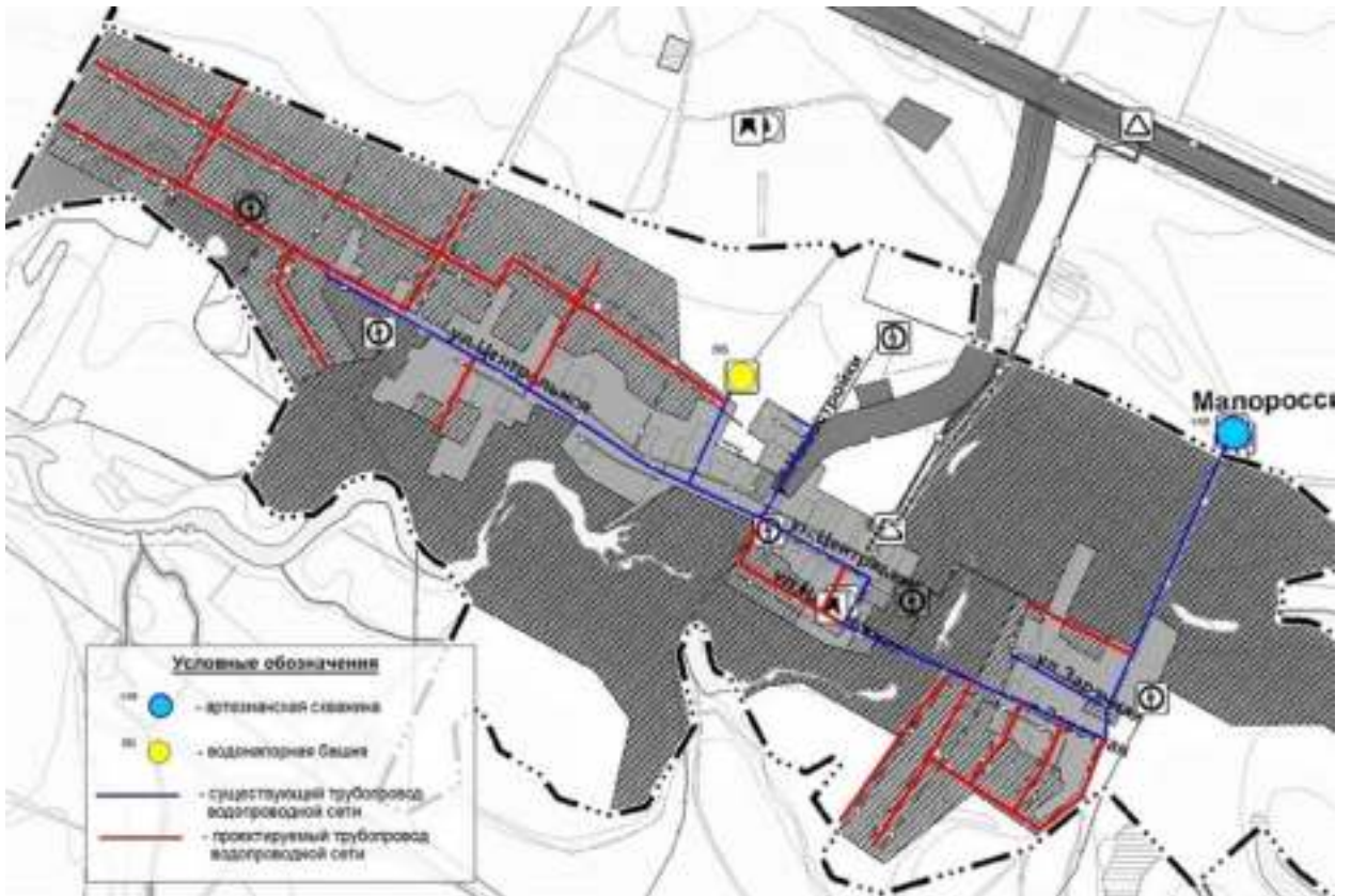
Рисунок 2.4.9.6 – Расположение существующих и перспективных объектов системы водоснабжения п. Малороссийский
