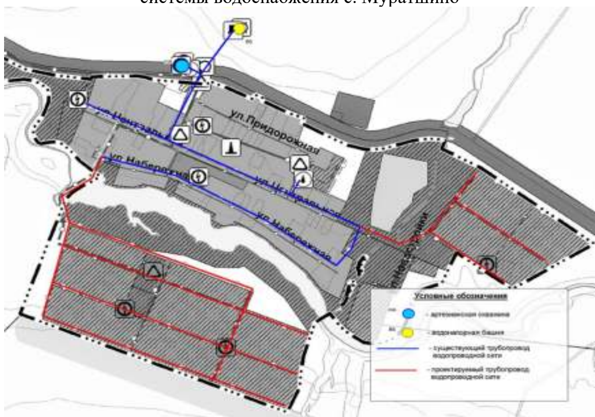
Рисунок 2.4.9.3 – Расположение существующих и перспективных объектов системы водоснабжения с. Таш-Кустьяново
