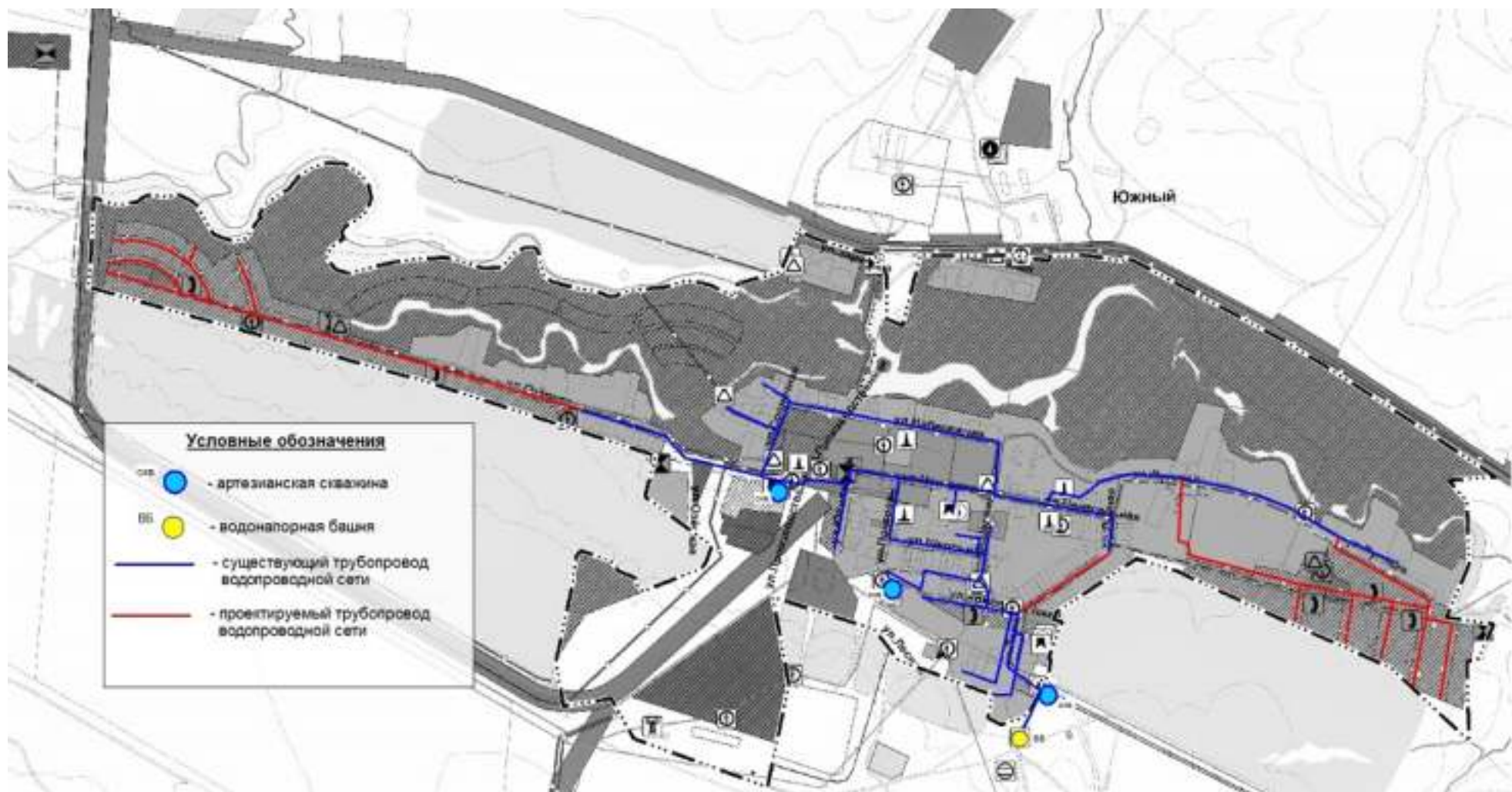
Рисунок 2.4.9.1 – Расположение существующих и перспективных объектов системы водоснабжения п. Южный
