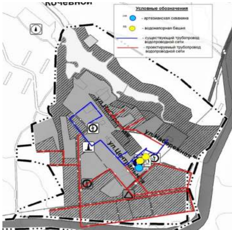
Рисунок 2.4.9.4 – Расположение существующих и перспективных объектов системы водоснабжения п. Кочевной
