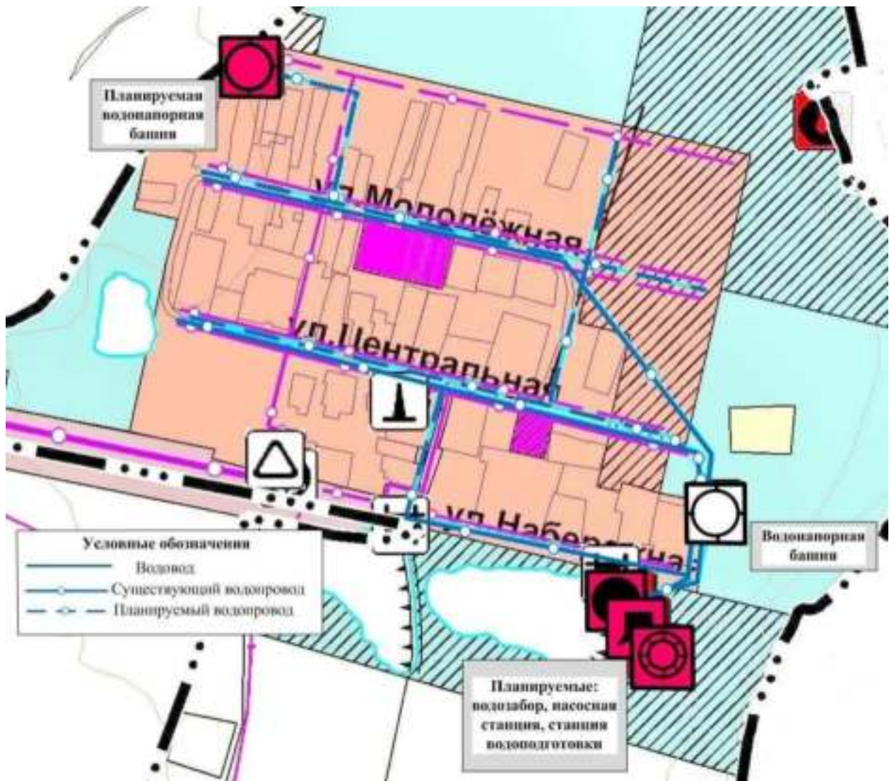
Рисунок 2.4.9.2 - Схема существующего и планируемого размещения объектов централизованной системы водоснабжения на территории посёлка Ледяйка
