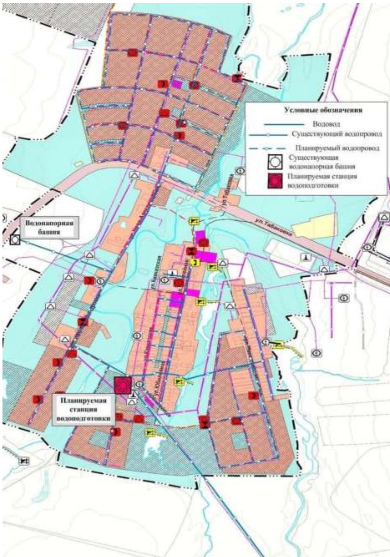
Рисунок 2.4.9.1 - Схема существующего и планируемого размещения объектов централизованной системы водоснабжения на территории села Мокша
