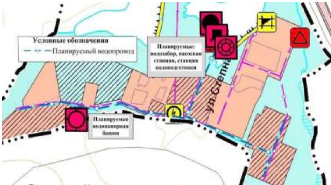
Рисунок 2.4.9.4 - План развития централизованной системы водоснабжения на территории посёлка Степной
