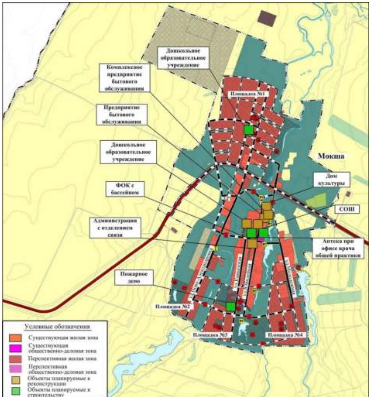
Рисунок 2.3.7.1 - Территория села Мокша с выделенными площадками под жилую зону и объектами перспективного строительства
