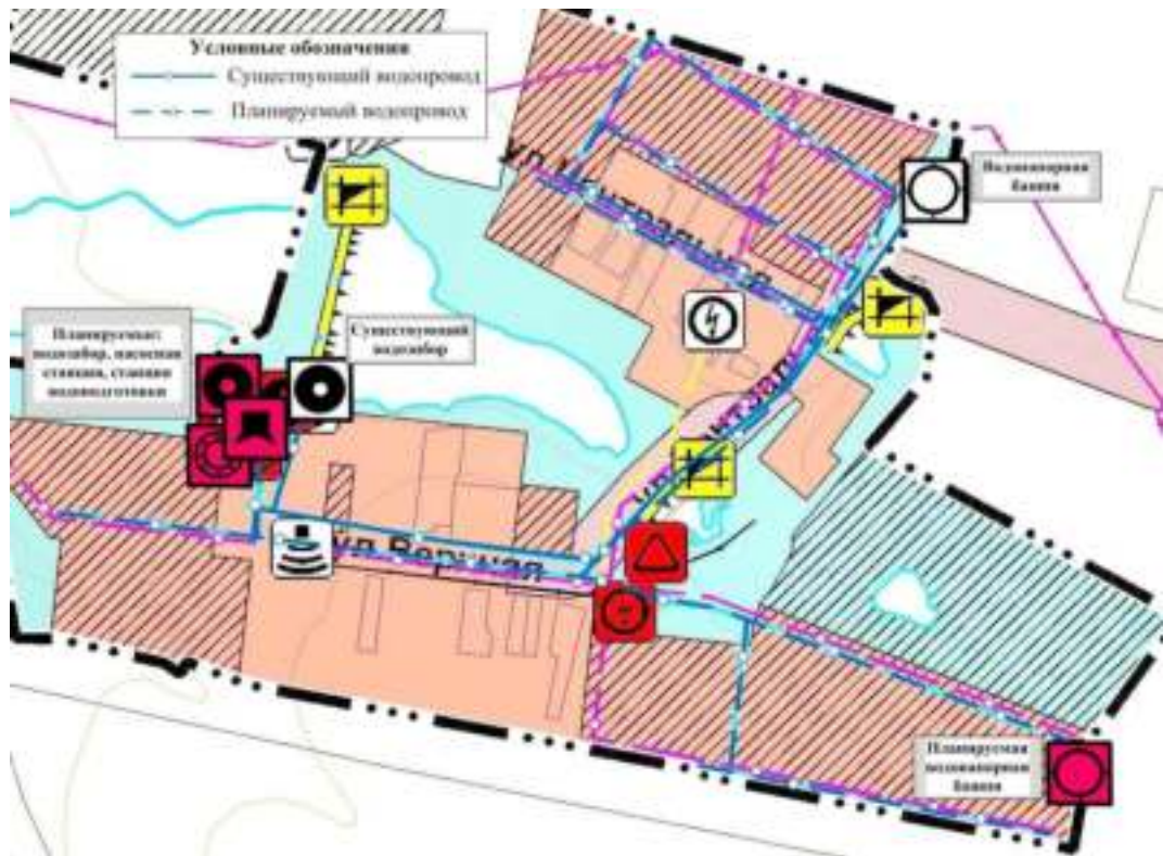
Рисунок 2.4.9.3 - Схема существующего и планируемого размещения объектов централизованной системы водоснабжения на территории посёлка Коммунар
